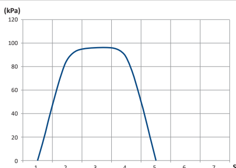
Diagramm des Druckanstiegs in einem Lufttaster mit Ø 32mm (wie das in diesem Katalog beschriebene Modell 66ZM5)
